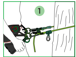
» Configuration à double sens
