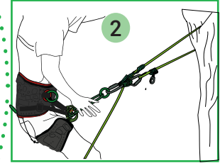
» Configuration simple avec poulie
