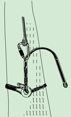
» ancrage au tronc
